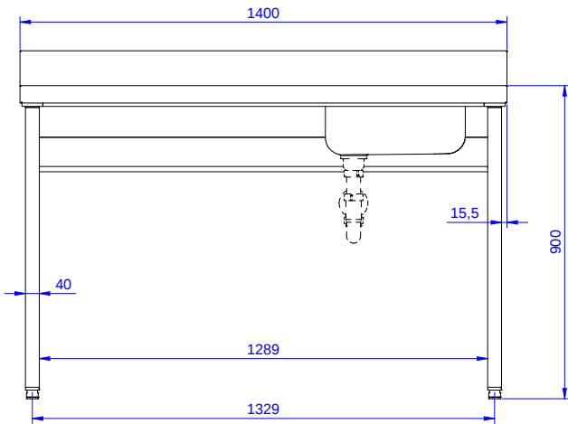
Sivulta
